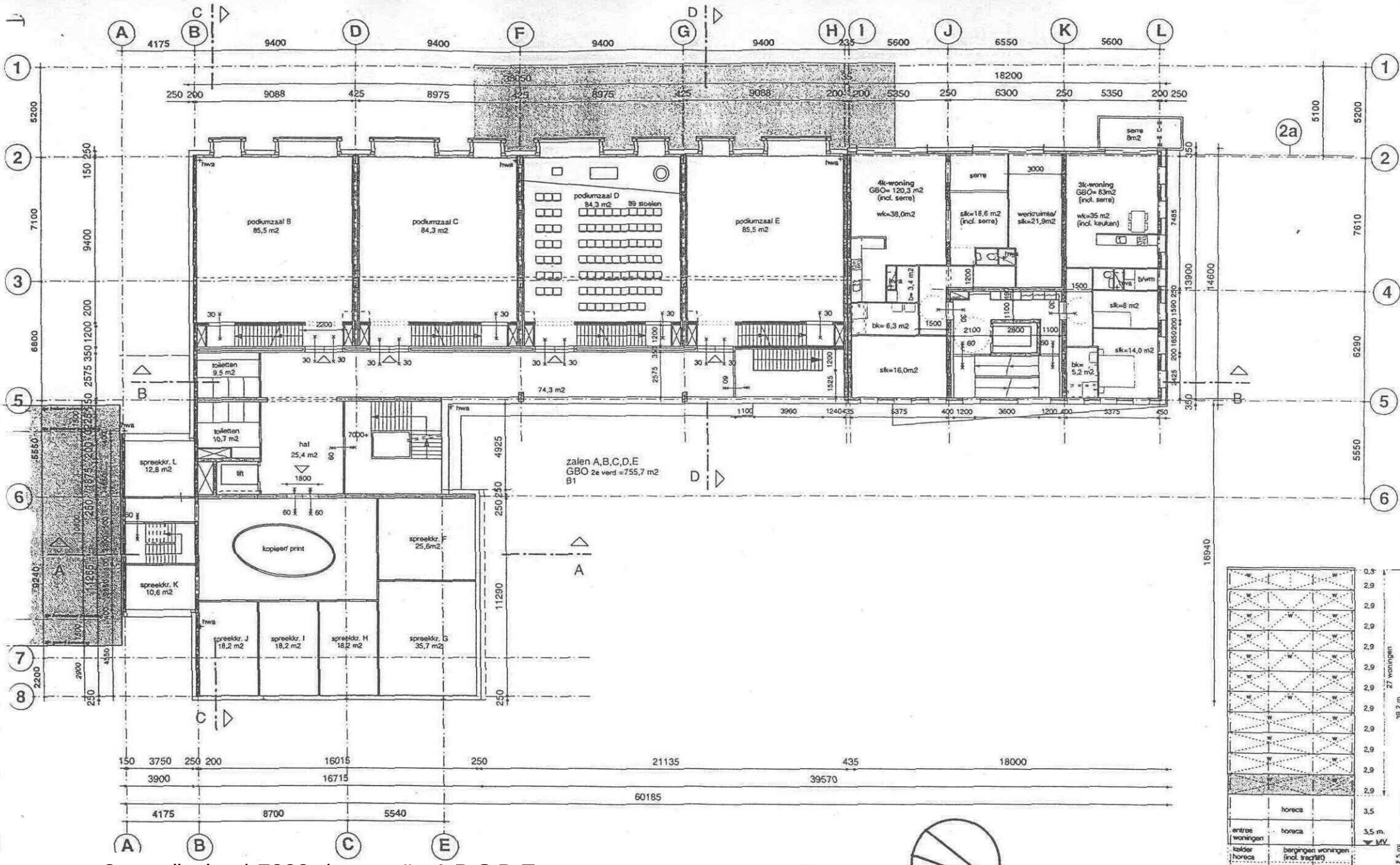
2e verdieping / 7000+ / traveeën A,B,C,D,E 2e verdieping / 7000+ / 27 woningen
