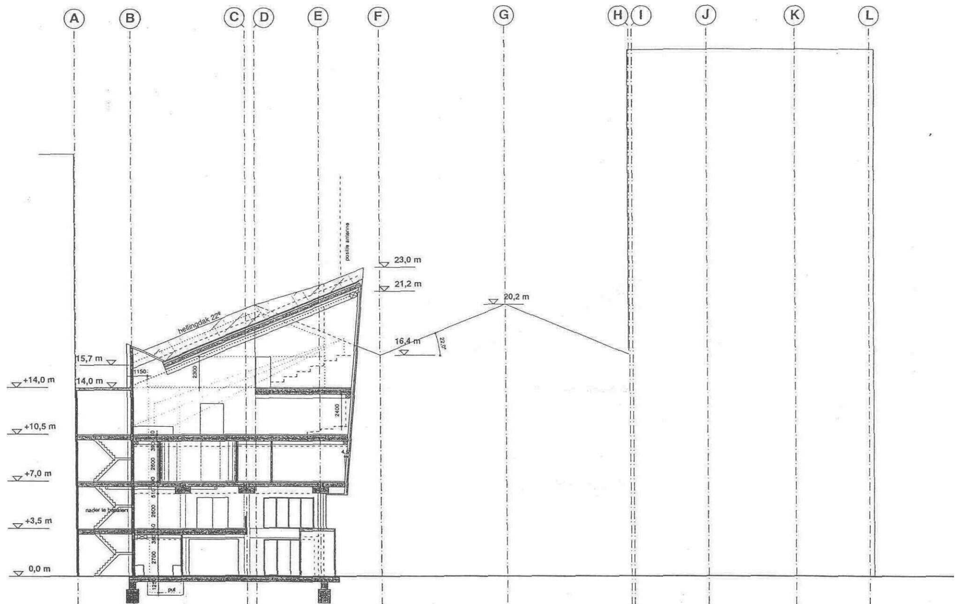
Dwars Doorsnede A-A
